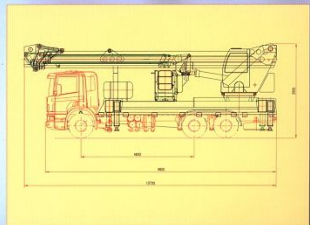
Ingombri su Strada - Road Overall Dimensions Dimensions Routieres - Dimensiones en Carretera
