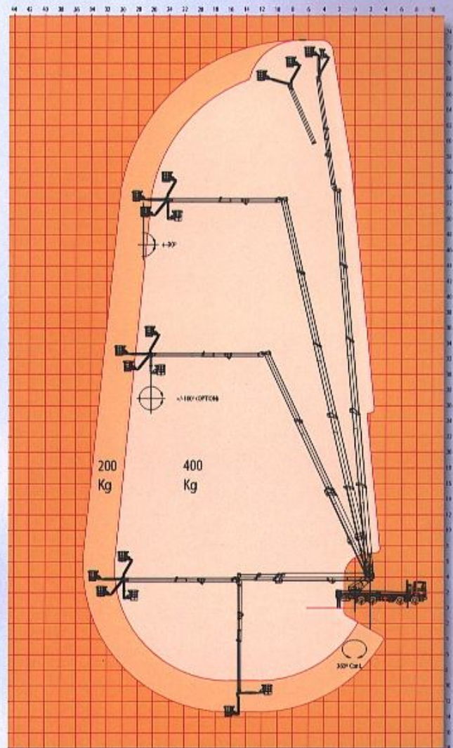
Campo di Lavoro - Work Range Diagram Champ de travail - Campo de Trabajo
