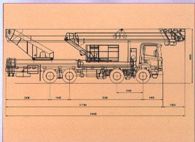
Ingombri su Strada - Road Overall Dimensions Dimensions Routières - Dimensiones en Carretera
